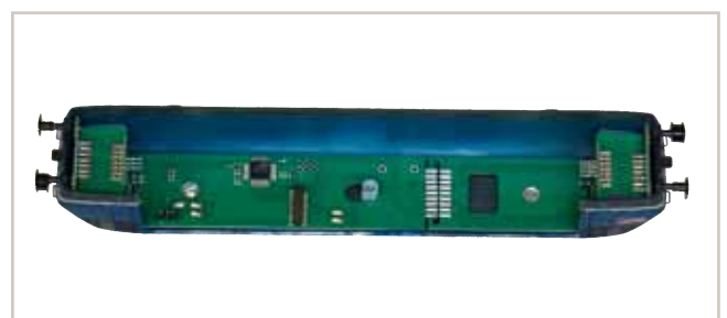
SBB Re 460/465 Elektronik Umbausatz
