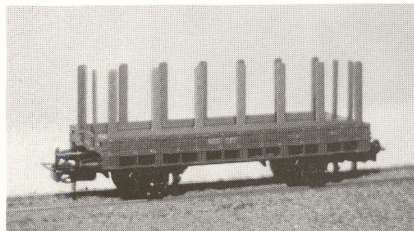
Nr. 360 Niederbordwagen Rungen abnehmbar
